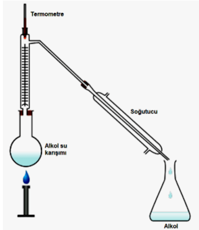
Alkol ve suyun damıtma ile ayrılması
