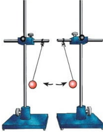
Aynı yüklü cisimler birbirini iter
