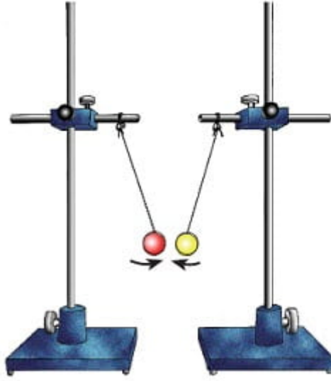
Zıt yüklü cisimler birbirini çeker
